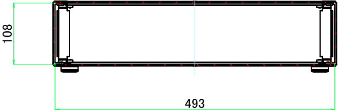
A-A ( 1 : 6.5 )
