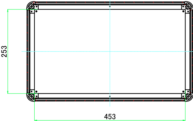
C-C ( 1 : 6.5 )
